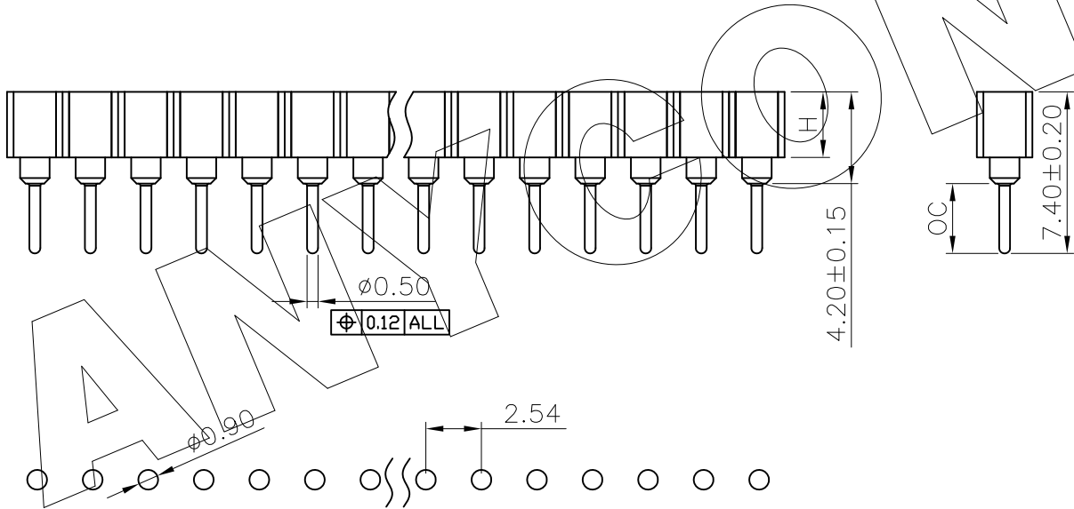
P.C.B LAYOUT
