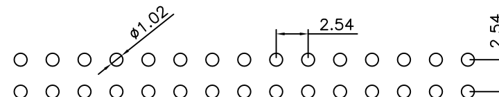
P.C.B LAYOUT
