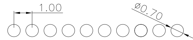
P.C.B LAYOUT
